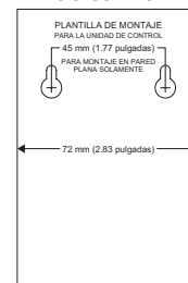
Plantilla de montaje de la unidad de control
